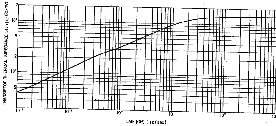
Fig.10 過渡熱抵抗
